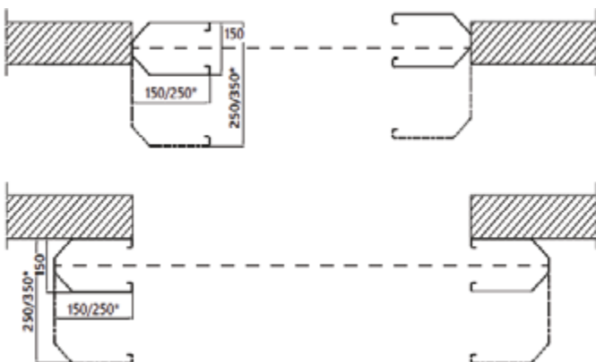
Detalles sujeción
